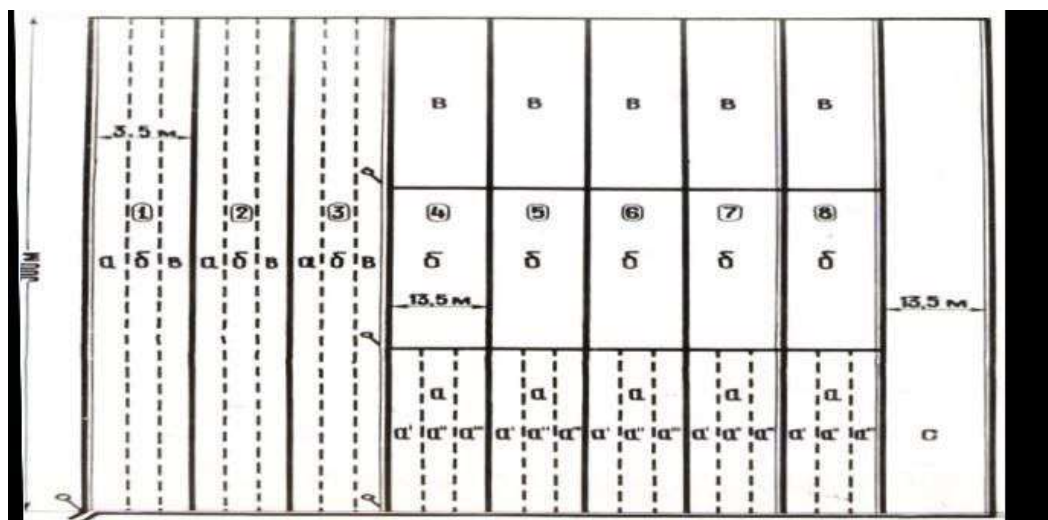
Рис.2. Схема опытного участка испытания водосберегающей технологии орошения 1 - делянка с полимером К-9 (малые струи), междурядье 0,9 м (борозда уплотнены); 2 — делянка с полимером к—9 (средние струи), междурядье 0,9 м (борозды уплотнены); 3 - делянка с полимером К—9 (большие струи), междурядье 0,3 м (борозда уплотнены); 4 - делянка с поролоновыми блокада 15x15x2,5 см, междурядье хлопчатника 0,45 м; 5 - делянка с полимерногрунтовыми блокада L=0,5 м, d =8 см, междурядье хлопчатника 0,45 м; б - делянка с поролоновыми блоками 15x17x2,5 см междурядие кукурузы 0,9 м; 7 - делянка с полимерногрунтовыми блоками L=0,5 м, d =8 см, междурядье кукурузы 0,3 м; 8 - делянка с поролоновыми блокада 15x12x 2,5 см междурядье посева люцерны 0,45 м; а, б, в, а', а', а''' - повторности; с - внутрипочвенное орошение.
