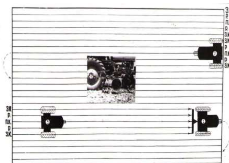
Рис.1 Поливной участок. Схема движения тракторов на поле для выполнения одноразового и двухразового уплотнения борозд.
