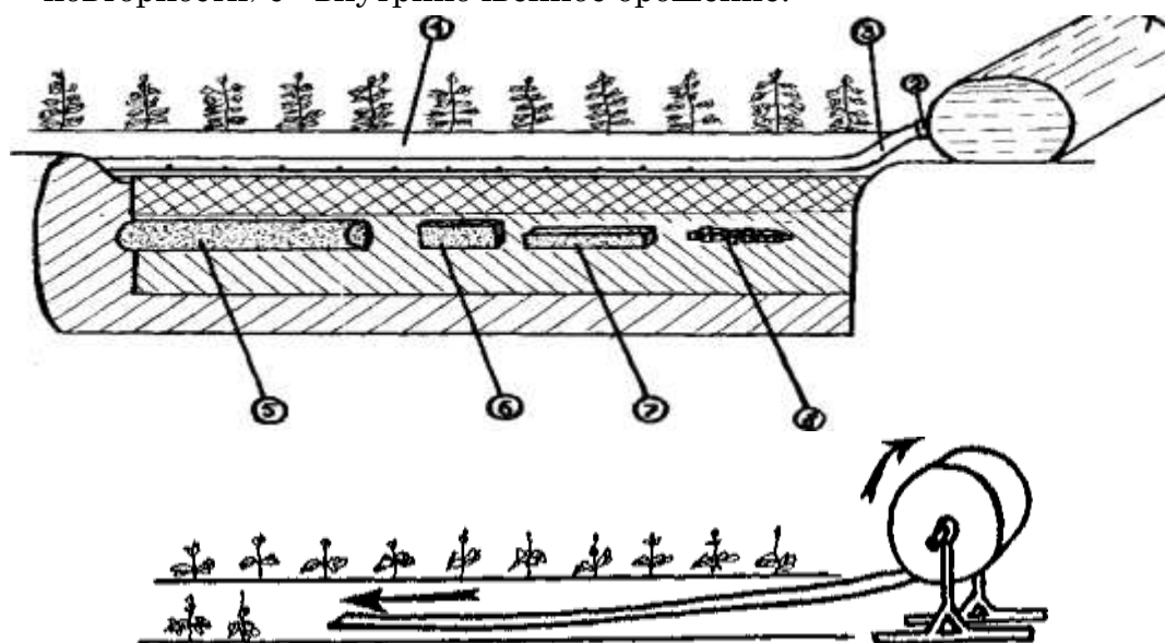
Рис.2.4. Блоки увлажнители под бороздами небольшой глубины, увлажняемые от шлангов малых диаметров с отверстиями 2 мм через 20 см 1 - гибкий шланг; 2 - водовыпуск в борозду; 3 - пленочный перфорированный шланг диаметром 5-7 см; 4 - поливная борозда глубиной 10-15 см; 5 - грунтополимерный блок -увлажнитель; 6,7,8 - блоки из поролона и обычной губки; 9 - раскладка малого шланга.
