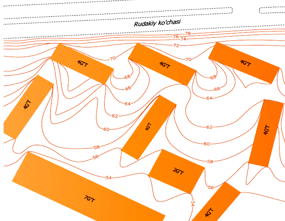
2-расм Рудакий кўчасидаги бинолар жойлашувига асосан шовқиннинг тарқалиш схемаси
